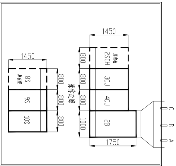
10kV 配电室平面布置图
